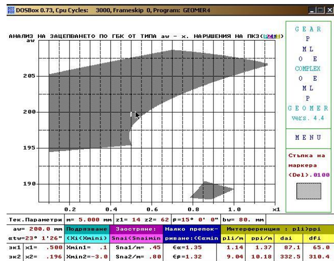
Фиг. 1 Блокиращ контур „a w x” m=5, z 1 =14, z 2 =62
